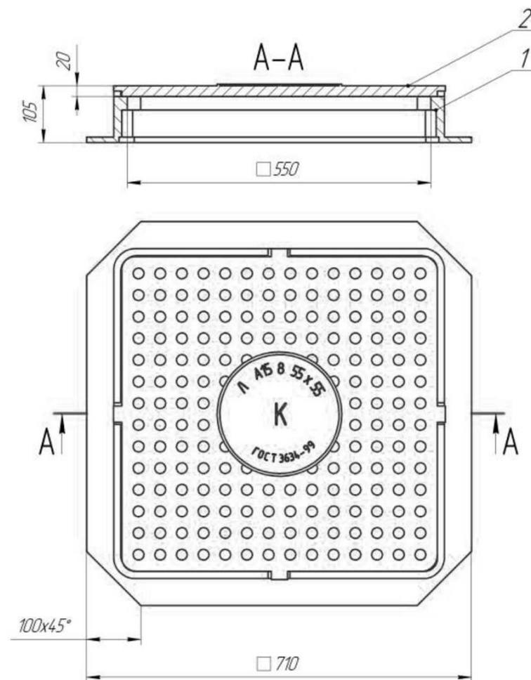
Рис. 1 Люк смотрового колодца лёгкий Л-А15-К-8-55х55.00-01 1. Корпус; 2. Крышка.
