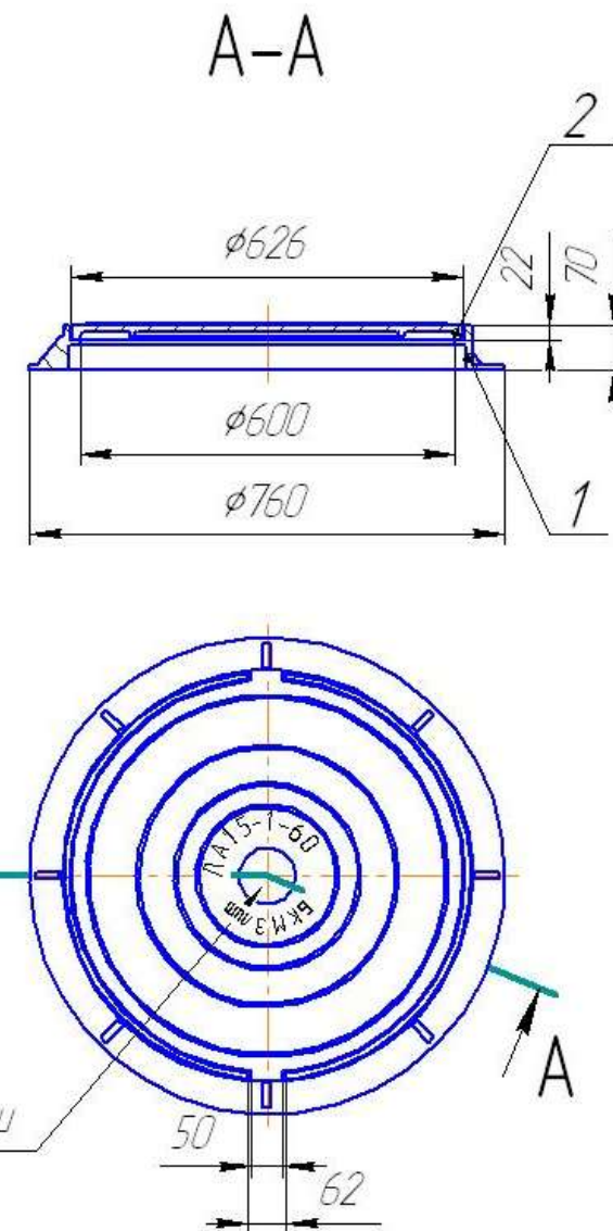
Рис.1 Люк смотрового колодца легкий Л-А15-1-60.00 1. Крышка; 2. Корпус.
